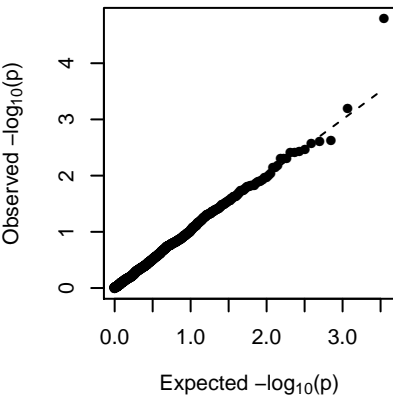
MEplum1 (1-dom-ref)
