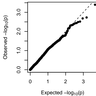
MEwhite (2-dom-ref)
