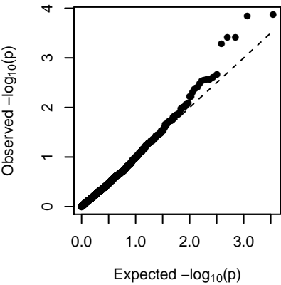
MEroyalblue (1-dom-ref)
