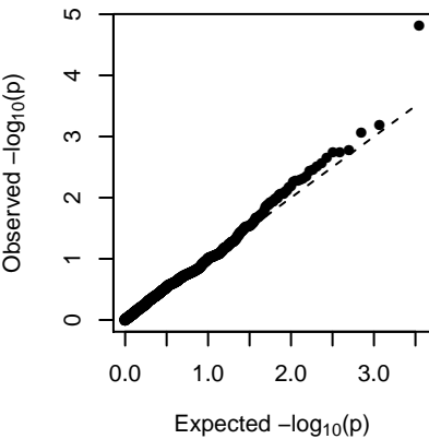
MEblack (1-dom-ref)
