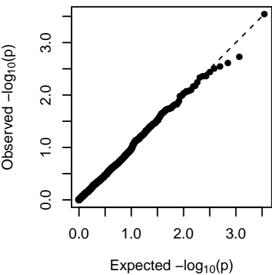
MEgreenyellow (1-dom-ref)
