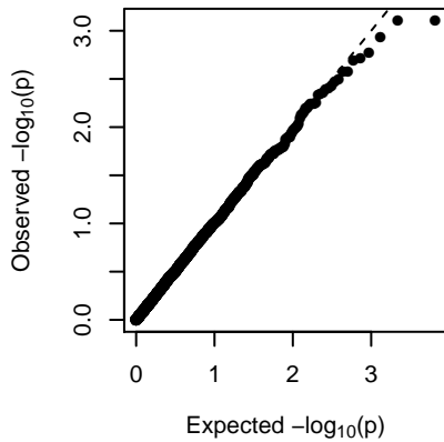
MEMagenta (general)
