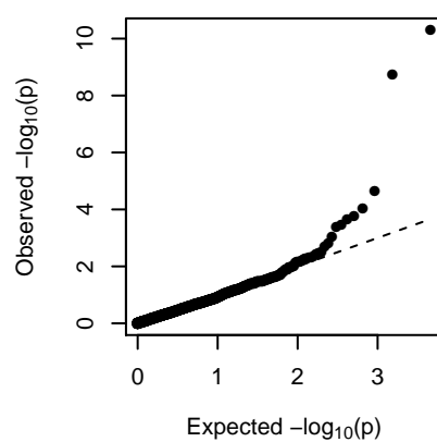
MEdarkorange (2-dom-ref)
