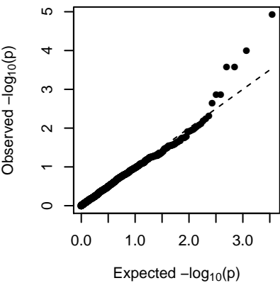
MEdarkturquoise (1-dom-ref)
