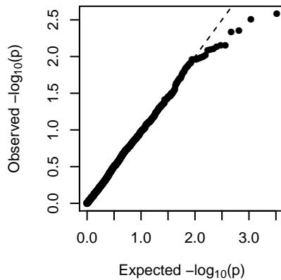
MEdarkmagenta (1-dom-alt)
