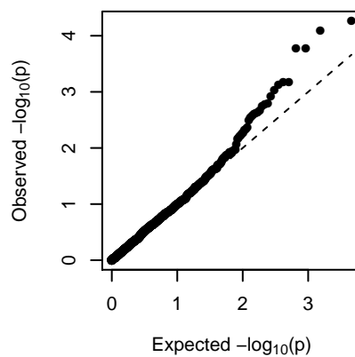
MEblack (2-dom-ref)
