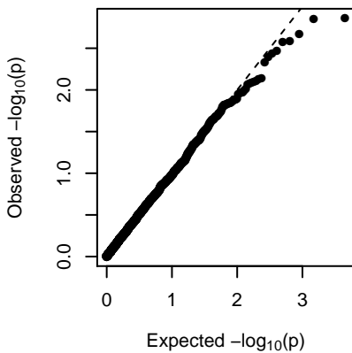
MEgreenyellow (2-dom-alt)
