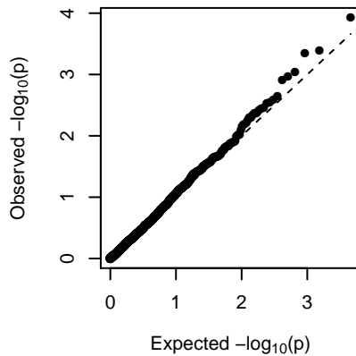
MEMagenta (2-dom-ref)
