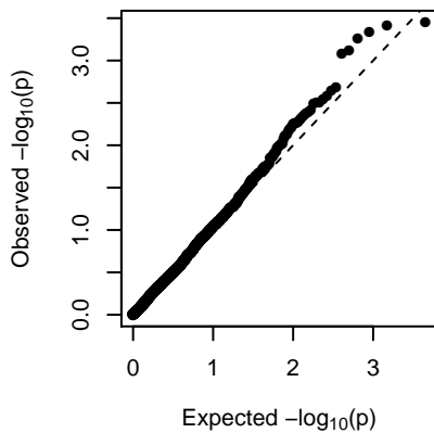
MEsienna3 (2-dom-alt)
