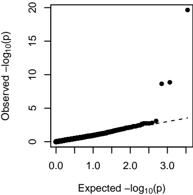
MEviolet (1-dom-ref)
