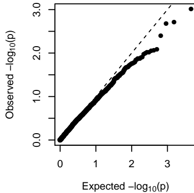
MEplum1 (2-dom-ref)
