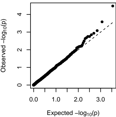
MEorangered4 (1-dom-ref)
