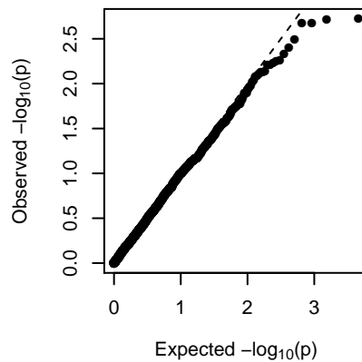
MEplum2 (2-dom-ref)
