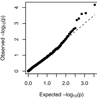
MEturquoise (1-dom-ref)
