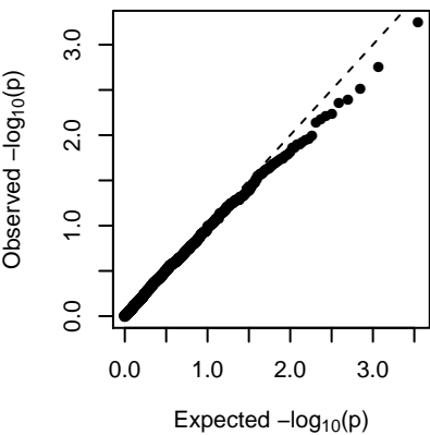
MEdarkslateblue (1-dom-ref)
