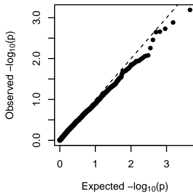
MEdarkgreen (2-dom-ref)
