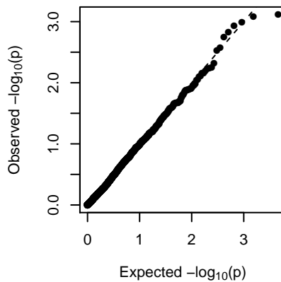
MEdarkorange2 (2-dom-ref)
