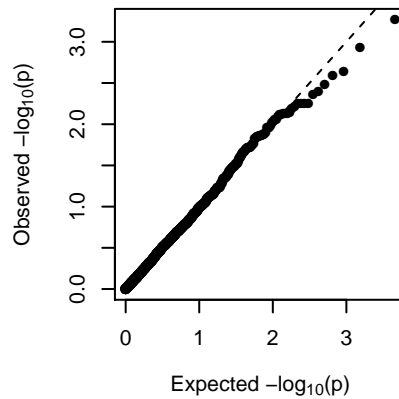
MEbrown (2-dom-ref)
