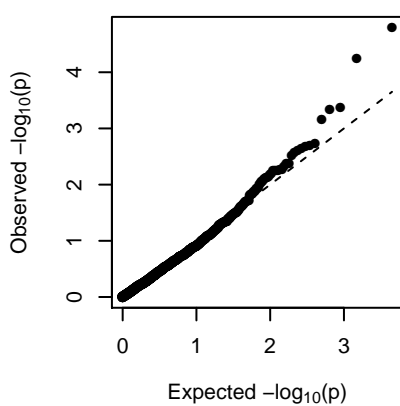
MEdarkorange (2-dom-alt)
