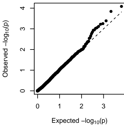
MEgreenyellow (general)
