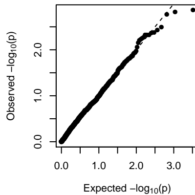
MEplum2 (1-dom-alt)
