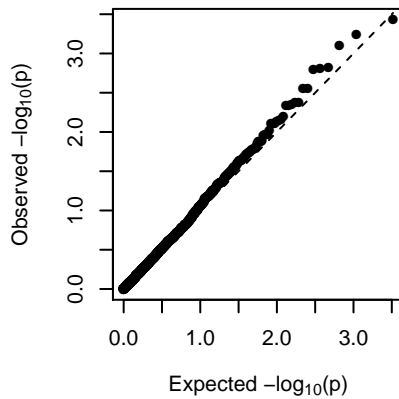
MEdarkred (1-dom-alt)
