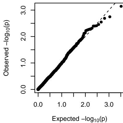
MEmidnightblue (1-dom-alt)
