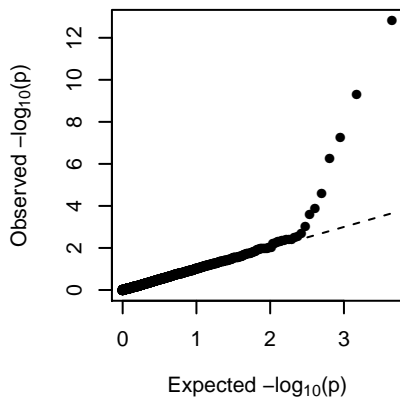
MEdarkturquoise (2-dom-alt)
