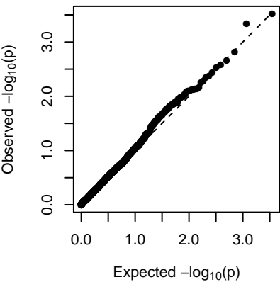
MEtan (1-dom-ref)
