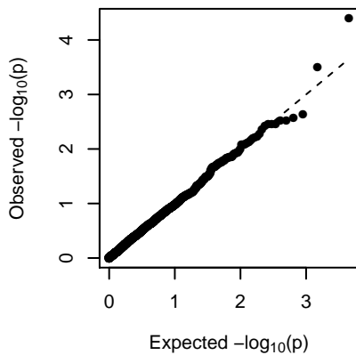
MEbrown4 (2-dom-alt)
