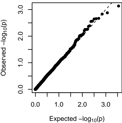
MElightyellow (1-dom-ref)
