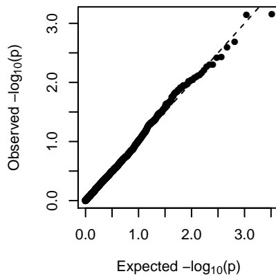
MEgreenyellow (1-dom-alt)
