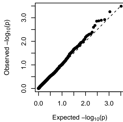
MEorangered4 (1-dom-alt)
