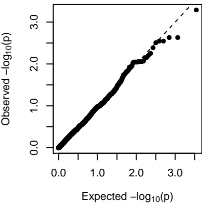
MEgrey (1-dom-ref)
