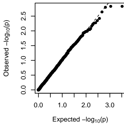
MEdarkgrey (1-dom-alt)
