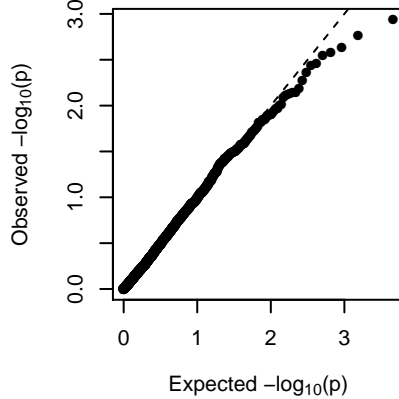
MEcyan (2-dom-ref)
