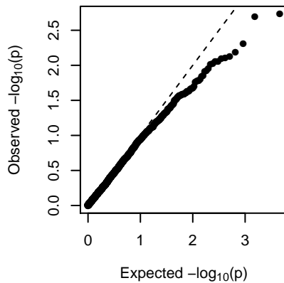
MEturquoise (2-dom-ref)
