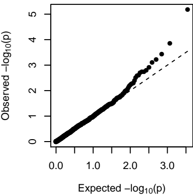
MEmediumpurple3 (1-dom-ref)
