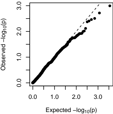
MElightgreen (1-dom-ref)
