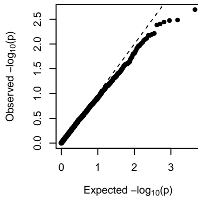
MEdarkmagenta (2-dom-ref)
