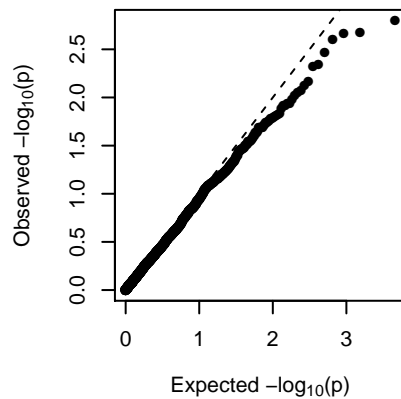
MEdarkslateblue (2-dom-ref)
