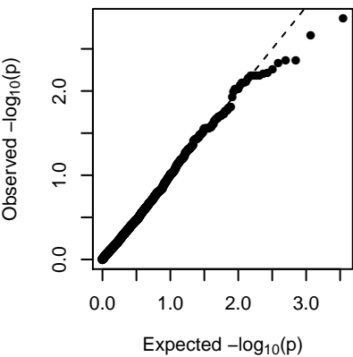
MEdarkgreen (1-dom-ref)
