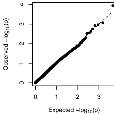
MEivory (2-dom-ref)
