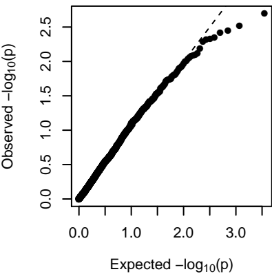
MEsaddlebrown (1-dom-ref)
