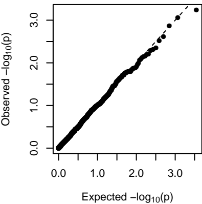
MEMagenta (1-dom-ref)
