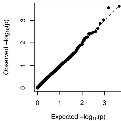
MElightgreen (2-dom-ref)
