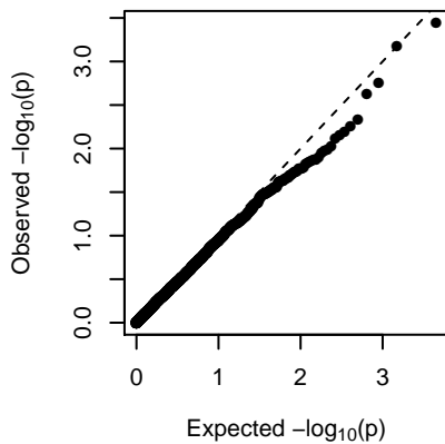
MEdarkred (2-dom-alt)
